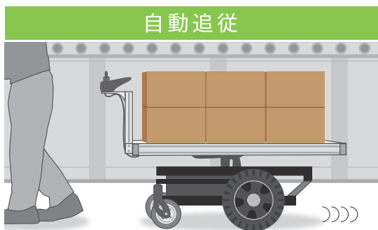
レーザーセンサで追従対象を認識
